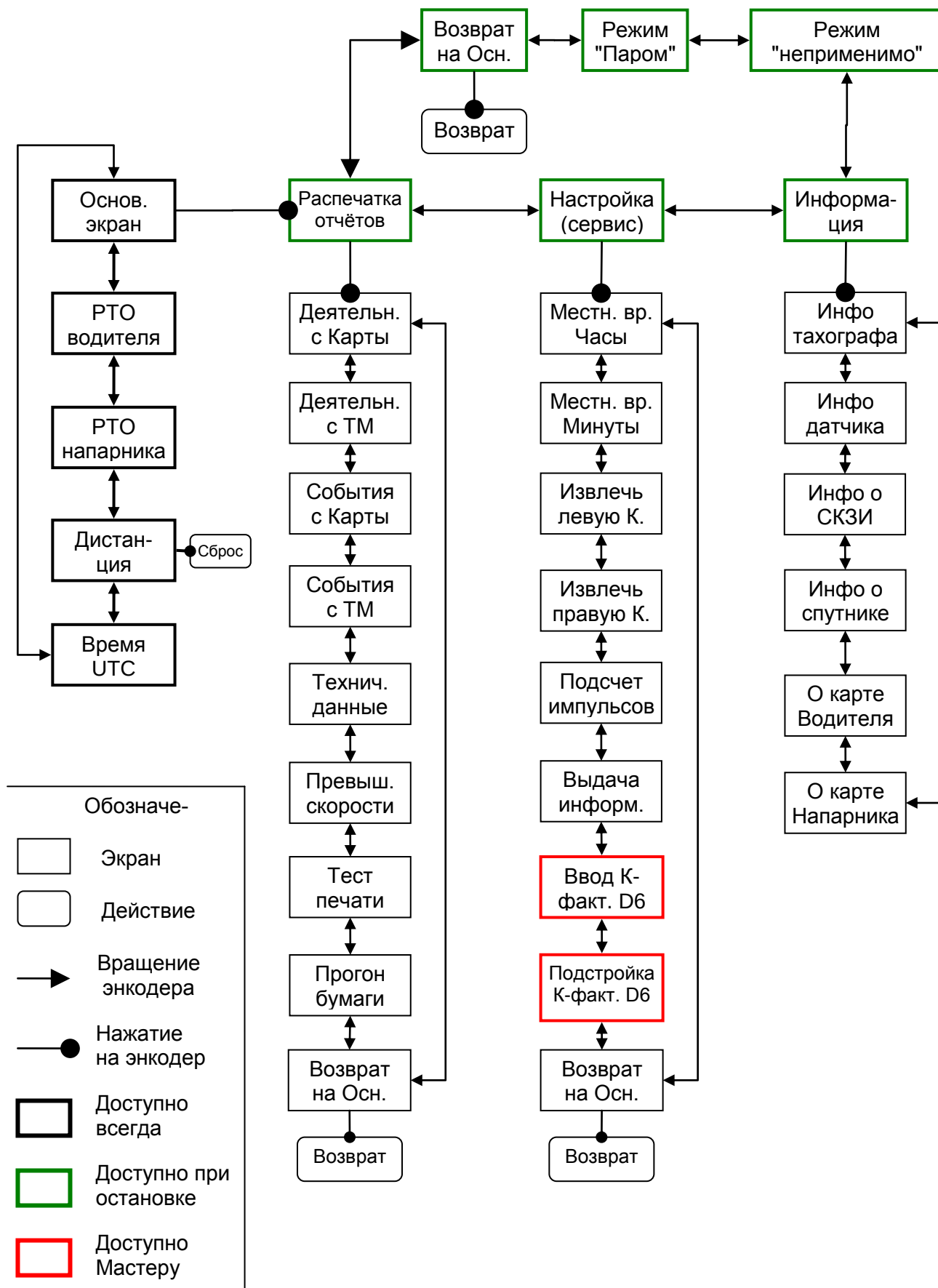
Рисунок 10. Схема меню тахографа ТЦА-02НК с версией ПО v.2.52
