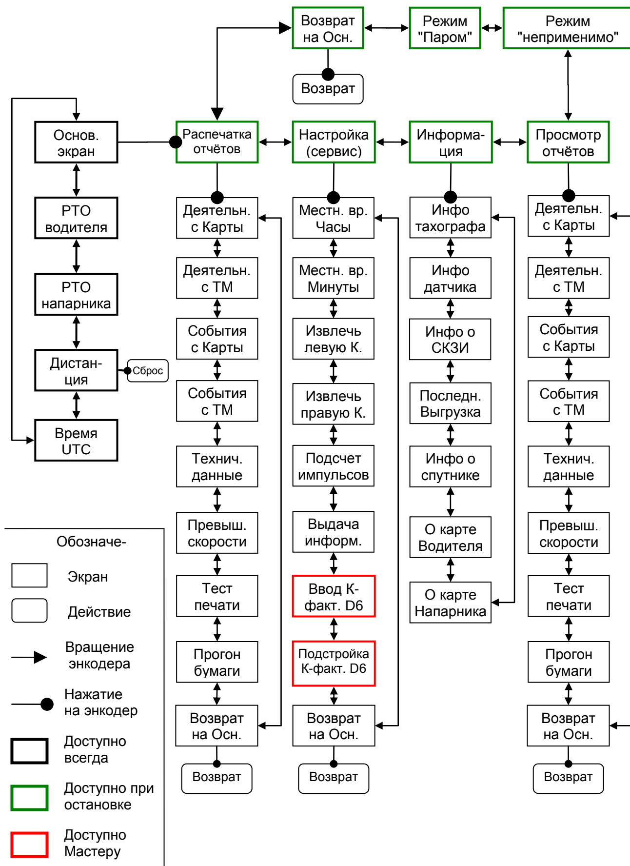
Рисунок 11. Схема меню тахографа ТЦА-02НК с версией ПО v.03.03
