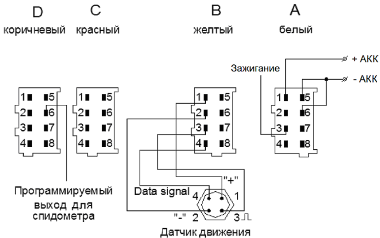
Рисунок 9. Схема подключения тахографа при использовании спидометра с программируемым входом
