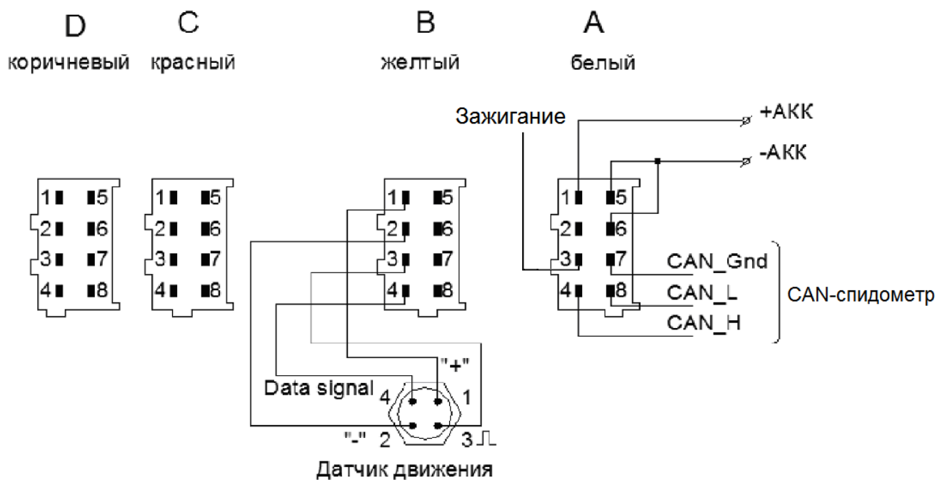
Рисунок 8. Схема подключения тахографа при использовании CAN-спидометра
