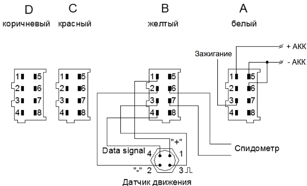
Рисунок 7. Схема подключения тахографа при использовании аналогового спидометра
