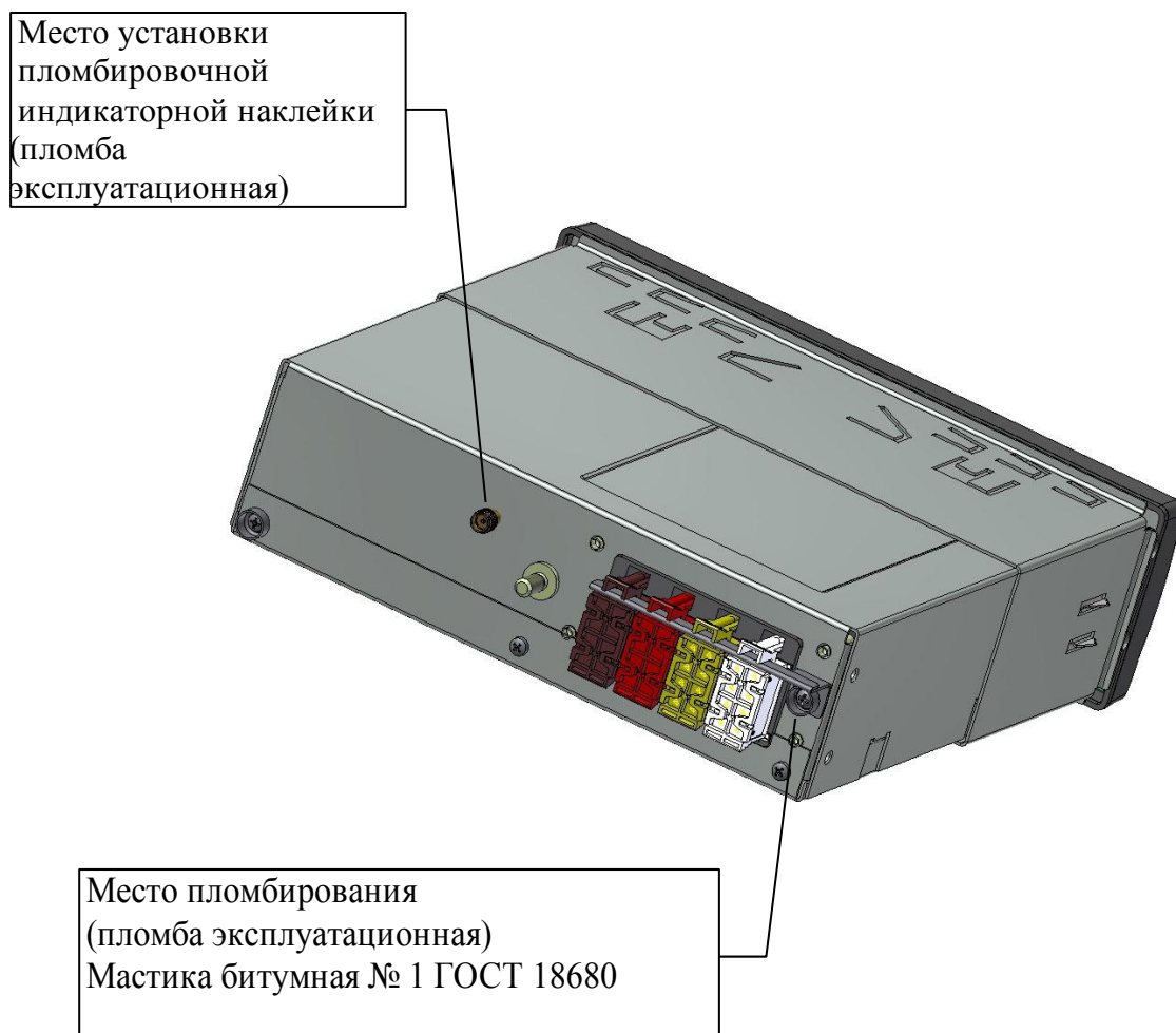
Рисунок 12. Пломба на заднем разъеме и разъеме антенны
